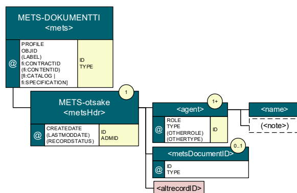
Kuva 3: Osa METS-profiilista
