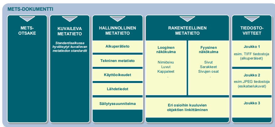
Kuva 2: METS-dokumentin rakenne
