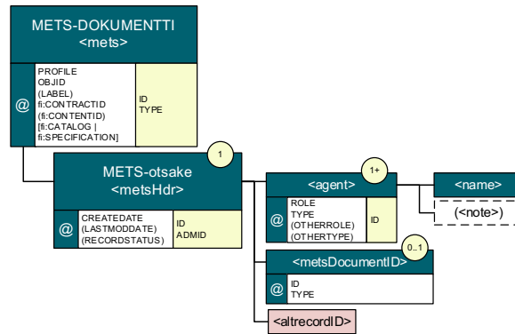
Kuva 3: Osa METS-profiilista
